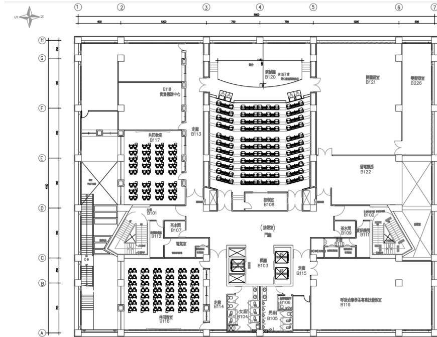
第一教學大樓 B1F 平面圖(FT)
